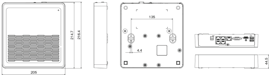
外形寸法図
