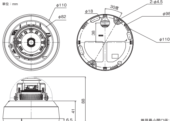
外形寸法図
