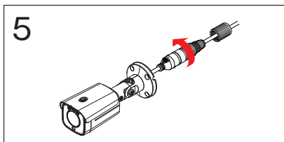
5 RJ45モジュラージャックとRJ45コネクタ保護カバーを接続し、回転して固定します。
