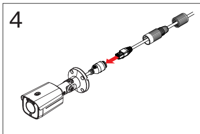
4 プラグポートとRJ45モジュラージャックを接続します。
