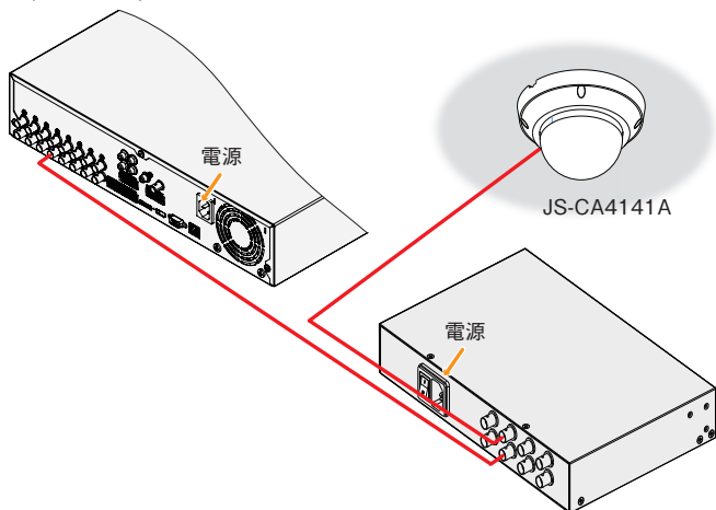
アナログHDカメラ専用PoC電源ユニット
