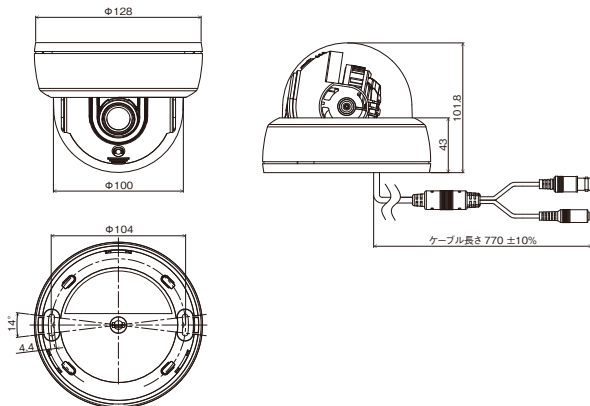
外形寸法図
