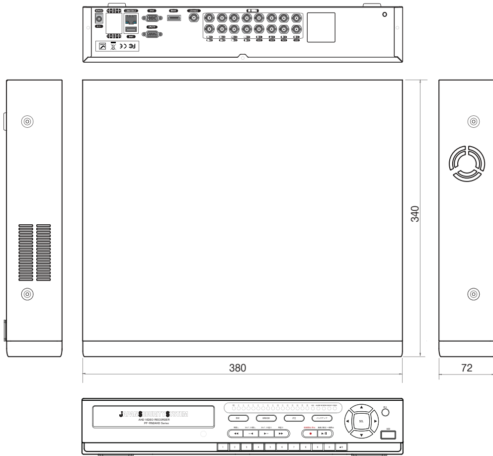
外形寸法図
