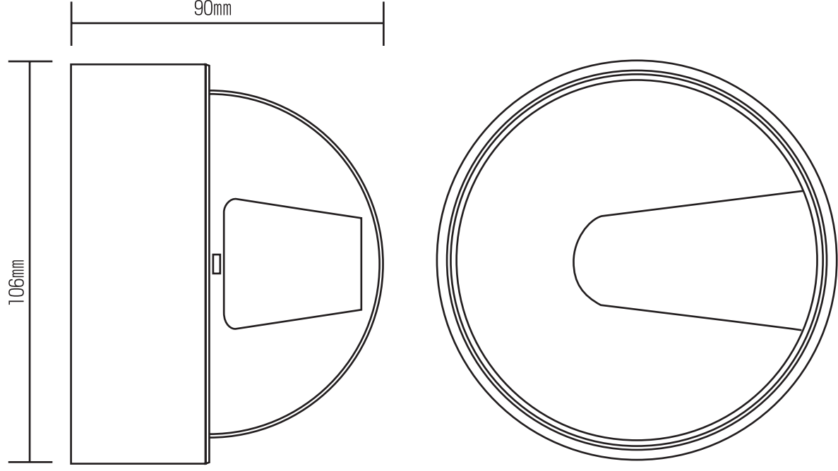
外形寸法図
