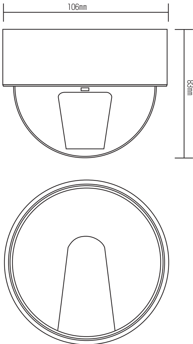
外形寸法図
